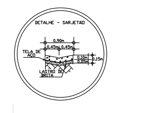
DETALHE - SARJETA
