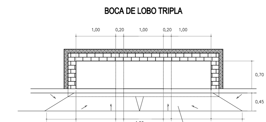
CORTE TRANSVERSAL
