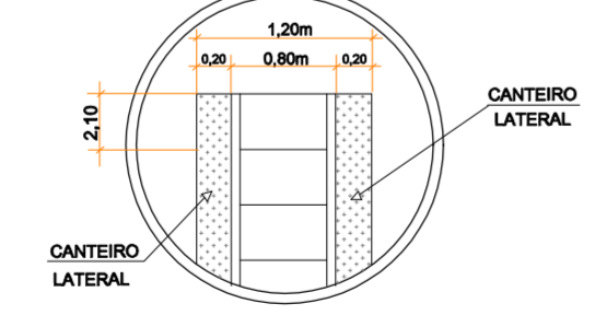
DETALHE - C-1 ESCADA HIDRÁULICA CORTE-1
