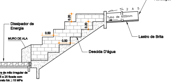
DETALHE - C-1 ESCADA HIDRÁULICA CORTE-1
