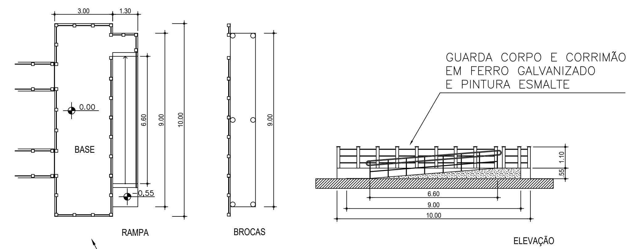
DETALHE DA RAMP A SER EXECUTADA AO LADO DA BASE
